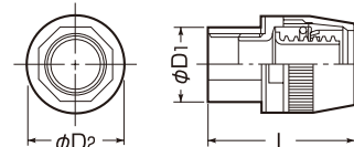
■マシンフレキ⇔厚鋼電線管(ねじ付)
