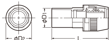
■マシンフレキ⇔薄鋼電線管(ねじ付)
