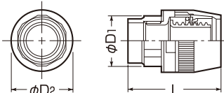
■マシンフレキ⇔VE管
