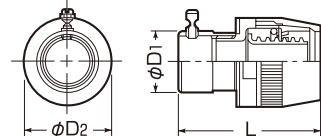
■マシンフレキ⇔厚鋼電線管(ねじ付)
