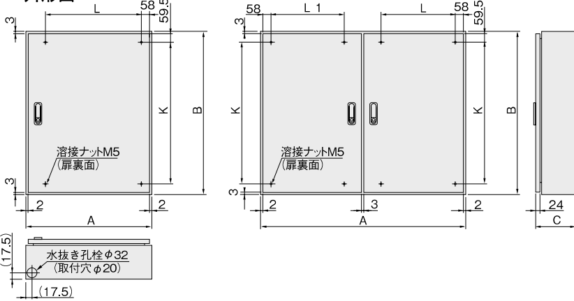
機器取付有効図 (扉)
