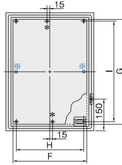
ボデー図
