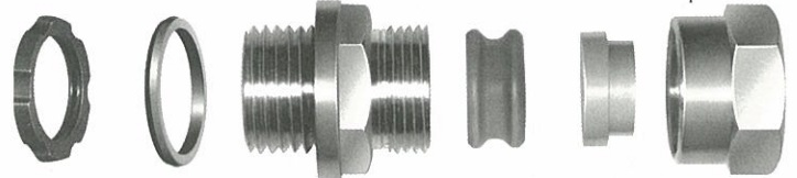
ロックナット (鋼製) ボディパッキン (NBR) ニップル ※(亜鉛) シールワッシング (NBR) テーパーワッシャ ※(ナイロン66) シメツケナット ※(亜鉛)
