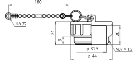
プラグキャップ：NJC-32-PCa
