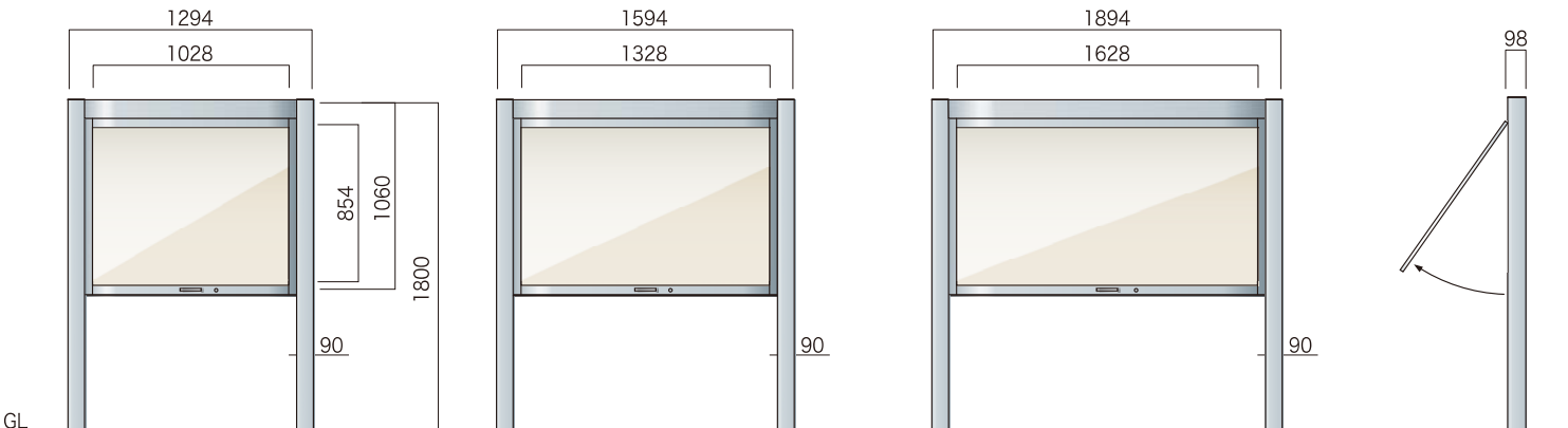
ダンパー付はね上げ式トビラ
