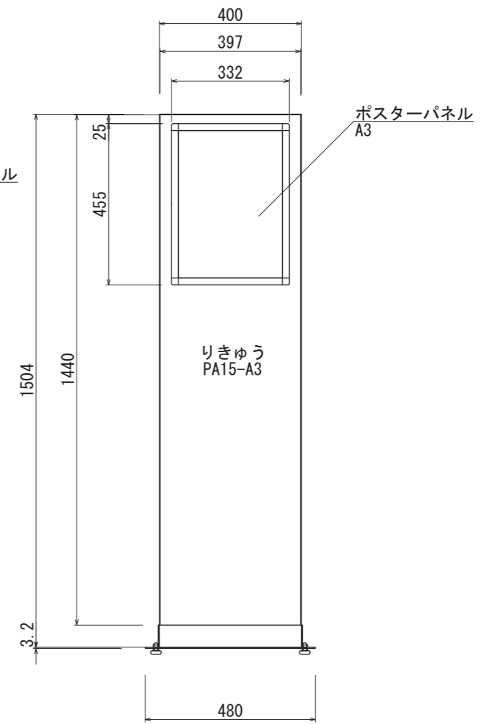
【正面図 S=1:15】
