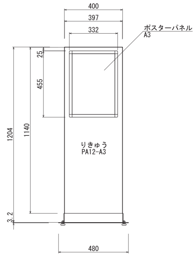
【正面図 S=1:15】
