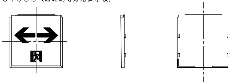
FK01038 (通路誘導灯用表示板)
