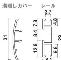
溝隠しカバー
