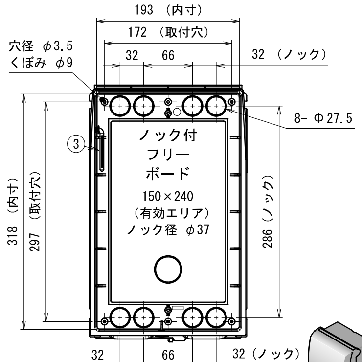
蓋無し参考図
