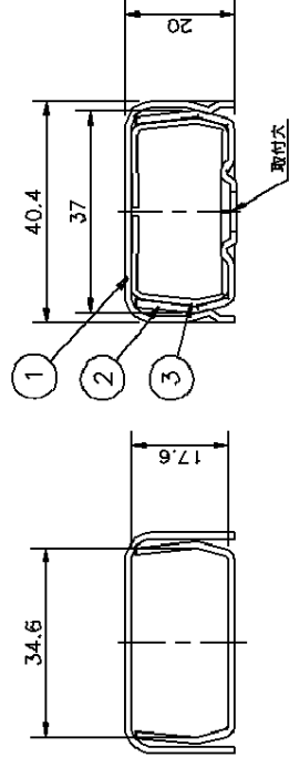
A-A断面
