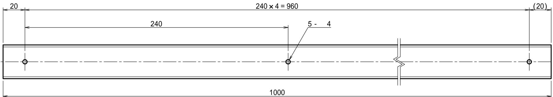
製品裏面釘穴図(1/2)
