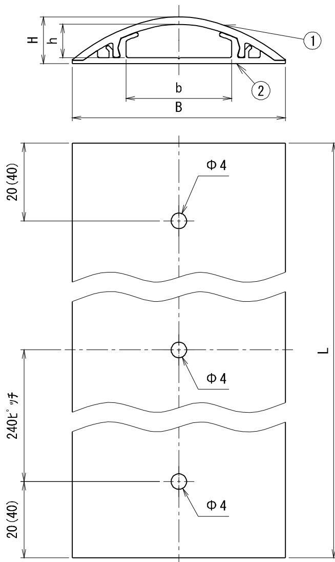
製品裏面釘穴図 ※ (40) 寸法はL寸法が2m品を示す。
