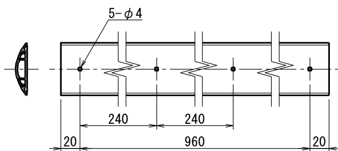
製品裏面釘穴図
