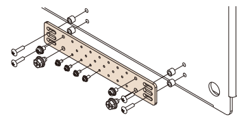
〔取付例：鉄製基板へ取り付けの場合〕
