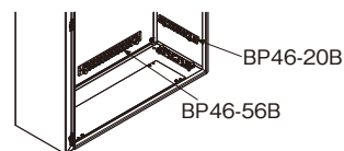
〔取付例2：キャビネット側面へ取り付けの場合〕
