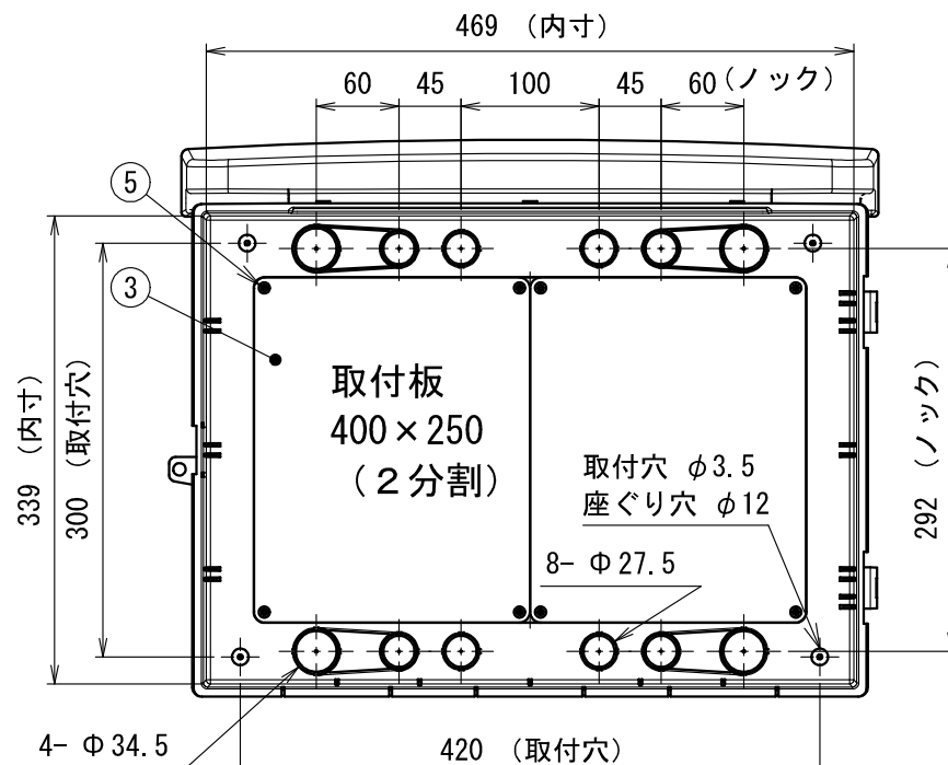
蓋無し参考図 1/6
