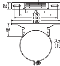
■POB-2型 器具取付溝(有効深さ20mm)
