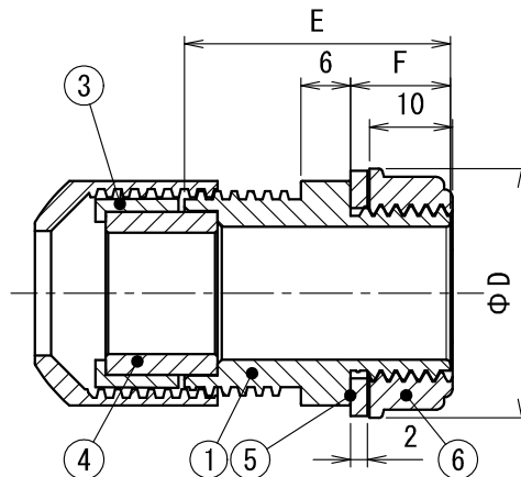
断面 A-A
