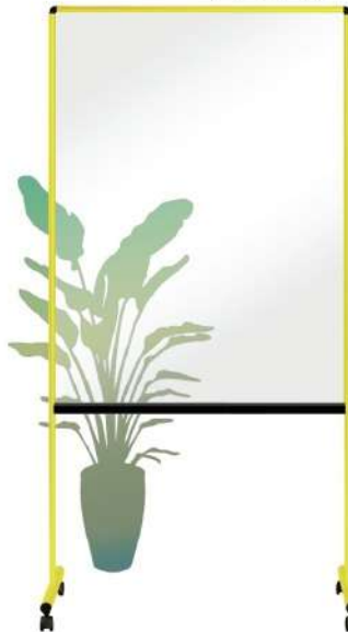
UDTP34N-Y 外形寸法/W939×D557×H1850 有効寸法/W883×H1170 質量 /14kg
