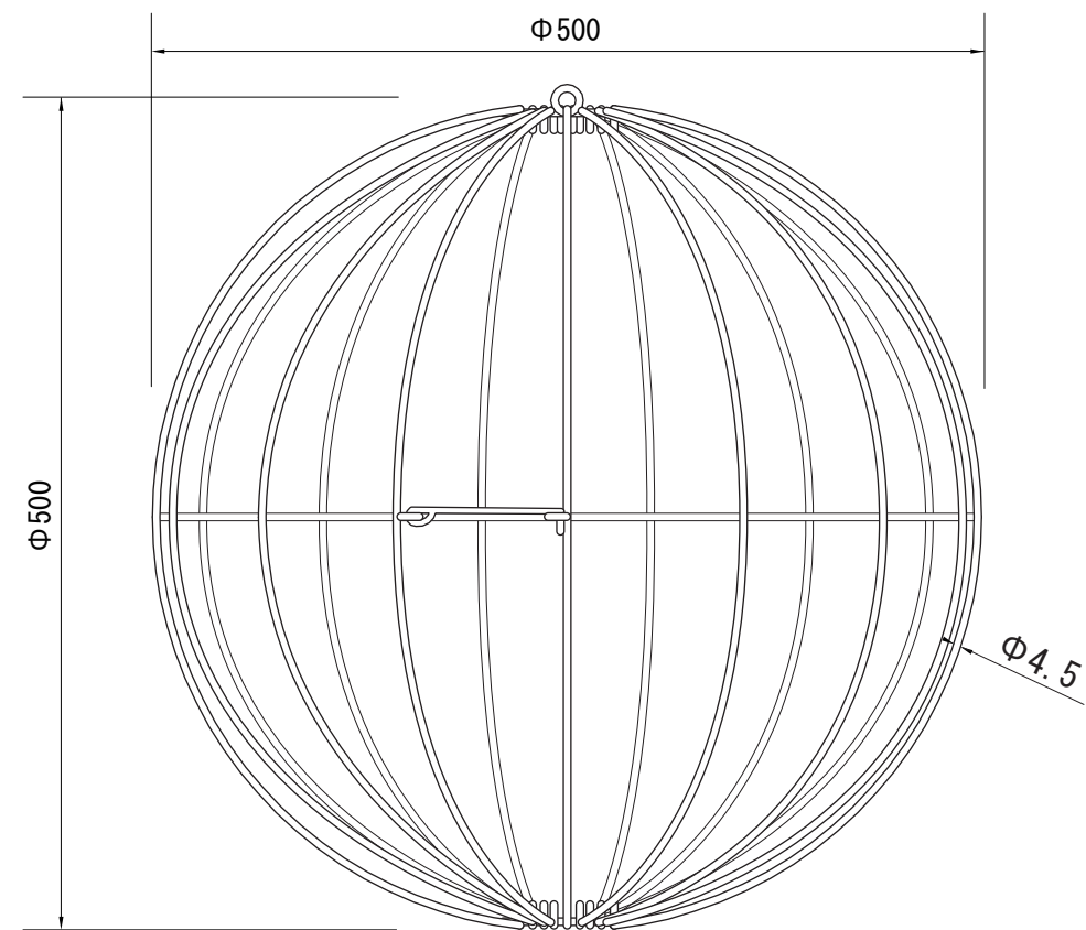
【正面図】
