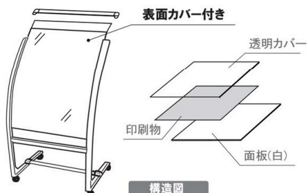
構造図
