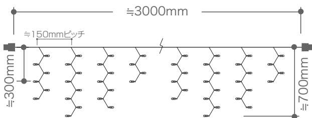
LEDプレイライトつらら ティンクル
