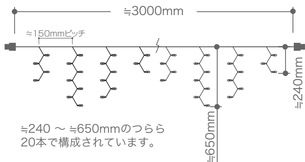
LEDプレイライトつらら フラッシュ
