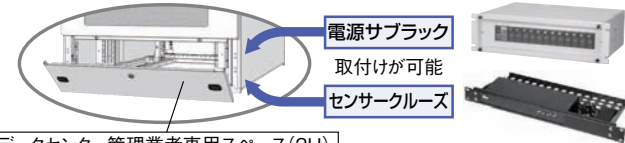
FSH100-720EN-1H (分割なし仕様) FSH100-720EN-2H (2分割仕様) FSH100-720EN-4H (4分割仕様)
