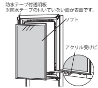
透明板の防水テープの内側に ソフトを合わせ、フレーム下辺の アクリル受けビスに載せてセットします。
