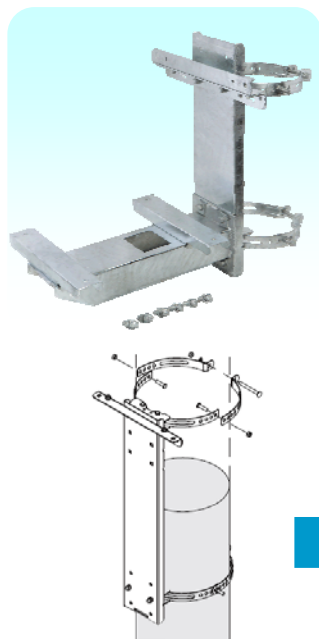
1. 本体のポール取付け
