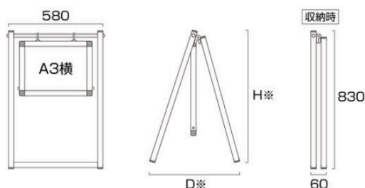
スイングサイン A3横 SWSAC-A3Y
