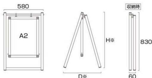
スイングサイン A2 SWSAC-A2
