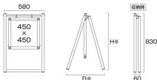
スイングサイン 450×450 SWSAC-450×450
