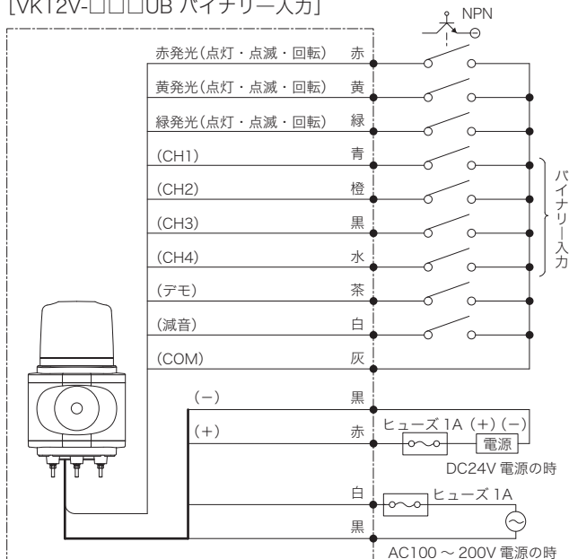
[VK12V-□□□UB バイナリー入力]
