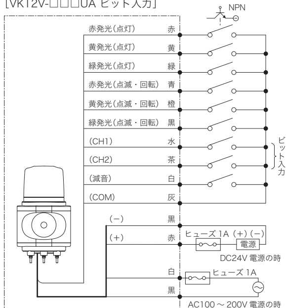
[VK12V-□□□UA ビット入力]
