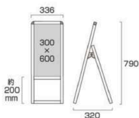
バリウススタンド看板 アルミ複合板 300×600片面 VASKAP-300×600K 12,430円(税込) シルバー
