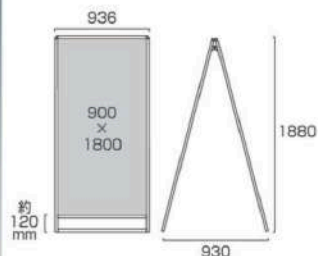
バリウススタンド看板 アルミ複合板 900×1800両面 VASKAP-900×1800R 52,140円(税込) シルバー
