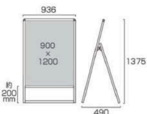
バリウススタンド看板 アルミ複合板 900×1200片面 VASKAP-900×1200K 29,480円(税込) シルバー
