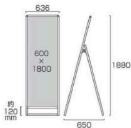
バリウスタンド看板 アルミ複合板 600×1800片面 VASKAP-600×1800K 32,780円(税込) シルバー
