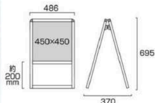
バリウススタンド看板 アルミ複合板 450×450両面 VASKAP-450×450R 17,380円(税込) シルバー
