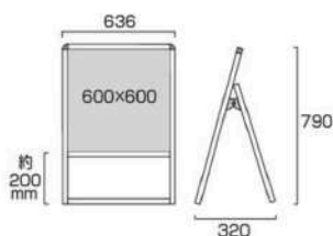
バリウススタンド看板 アルミ複合板 600×600片面 VASKAP-600×600K 14,960円(税込) シルバー
