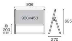
バリウスタンド看板 アルミ複合板 900×450片面 VASKAP-900×450K 16,280円(税込) シルバー
