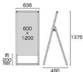
バリウススタンド看板 アルミ複合板 600×1200片面 VASKAP-600×1200K 21,560円(税込) シルバー
