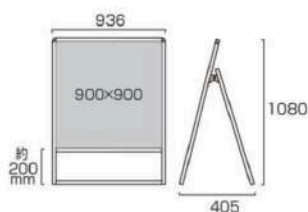
バリウススタンド看板 アルミ複合板 900×900片面 VASKAP-900×900K 21,560円(税込) シルバー
