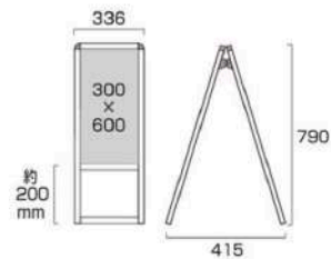
バリウススタンド看板 アルミ複合板 300×600両面 VASKAP-300×600R 16,060円(税込) シルバー
