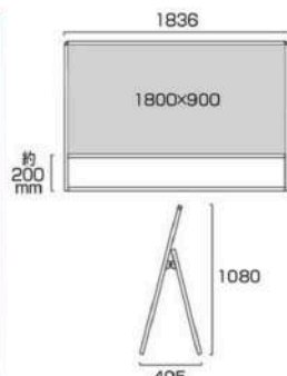
バリウススタンド看板 アルミ複合板 1800×900片面 VASKAP-1800×900K 39,820円(税込) シルバー
