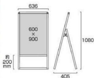
バリウススタンド看板 アルミ複合板 600×900片面 VASKAP-600×900K 18,040円(税込) シルバー
