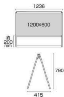
バリウススタンド看板 アルミ複合板 1200×600両面 VASKAP-1200×600R 38,720円(税込) シルバー
