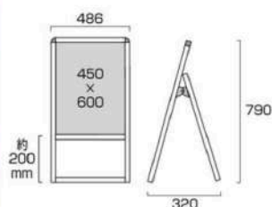
バリウススタンド看板 アルミ複合板 450×600片面 VASKAP-450×600K 13,420円(税込) シルバー
