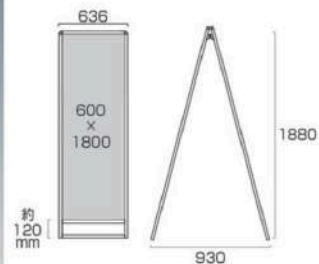
バリウスタンド看板 アルミ複合板 600×1800両面 VASKAP-600×1800R 44,660円(税込) シルバー
