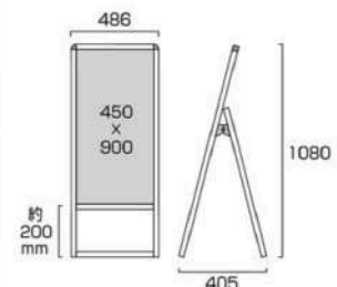
バリウススタンド看板 アルミ複合板 450×900片面 VASKAP-450×900K 15,180円(税込) シルバー
