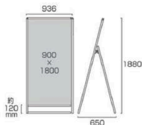
バリウススタンド看板 アルミ複合板 900×1800片面 VASKAP-900×1800K 38,720円(税込) シルバー
