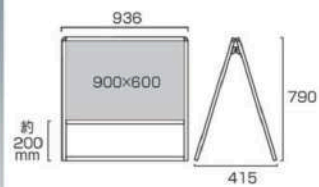
バリウスタンド看板 アルミ複合板 900×600両面 VASKAP-900×600R 29,480円(税込) シルバー
