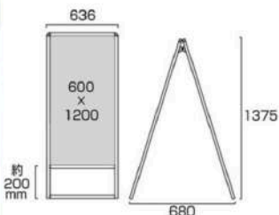
バリウススタンド看板 アルミ複合板 600×1200両面 VASKAP-600×1200R 36,520円(税込) シルバー
