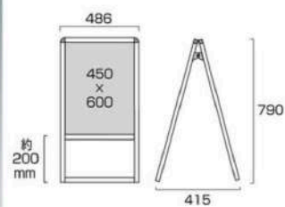
バリウススタンド看板 アルミ複合板 450×600両面 VASKAP-450×600R 20,240円(税込) シルバー
