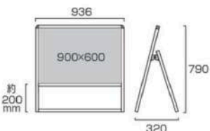
バリウスタンド看板 アルミ複合板 900×600片面 VASKAP-900×600K 19,140円(税込) シルバー
