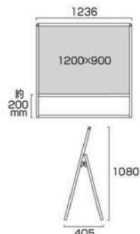
バリウススタンド看板 アルミ複合板 1200×900片面 VASKAP-1200×900K 30,580円(税込) シルバー
