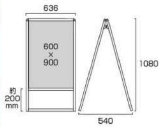
バリウススタンド看板 アルミ複合板 600×900両面 VASKAP-600×900R 27,280円(税込) シルバー
