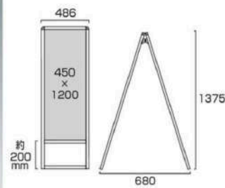
バリウススタンド看板 アルミ複合板 450×1200両面 VASKAP-450×1200R 27,280円(税込) シルバー
