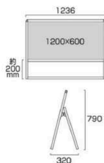
バリウススタンド看板 アルミ複合板 1200×600片面 VASKAP-1200×600K 22,660円(税込) シルバー
