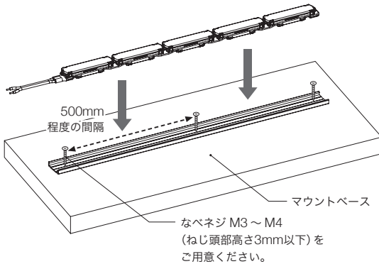
図2 直線施工する場合
