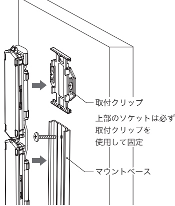
図5 垂直な壁や傾斜面へ設置する場合
