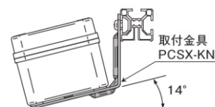
〔取付例〕
