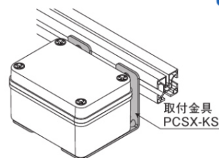
〔取付例〕
