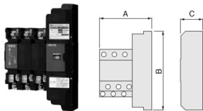
DS73MC 3P 75A
