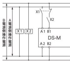
〔制御回路の一例〕
