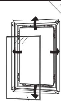
防水テープ付透明板
