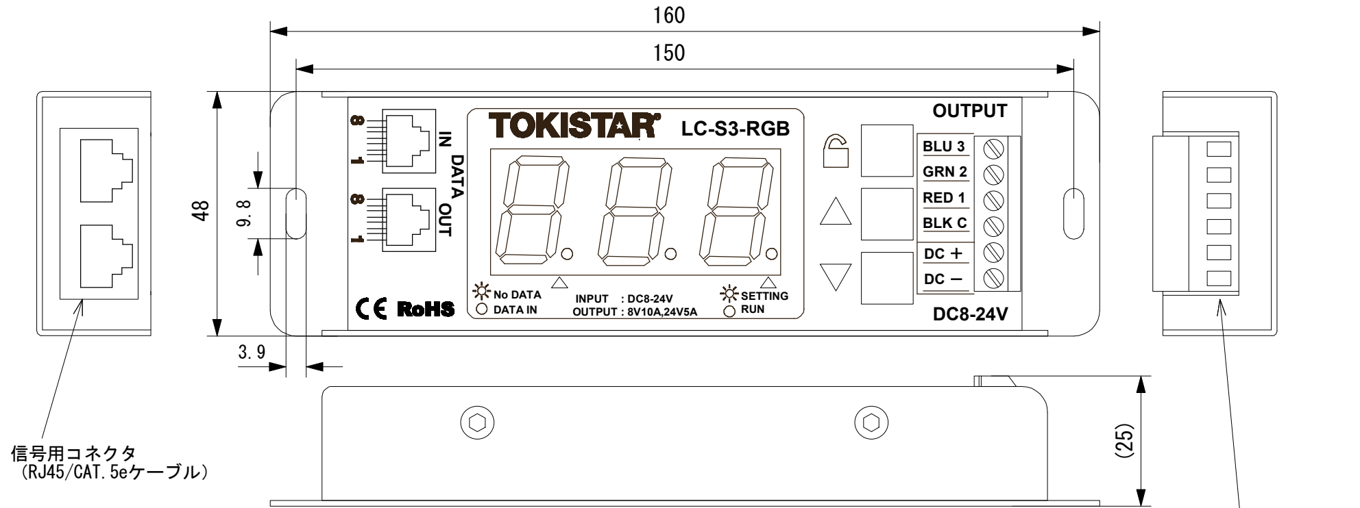
出力端子台 適合電線径 : AWG20~AWG14 (0.5~2.0sq)
