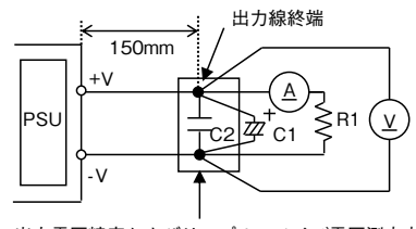
測定回路図
