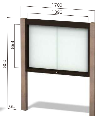
RGP-1510 照明なし ガラス引違いタイプ 設計価格 ¥367,400(外税)
