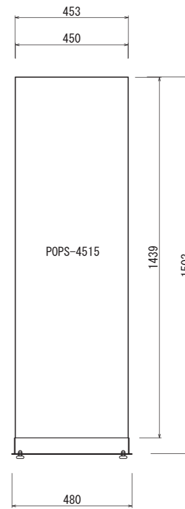
【正面図 S=1:15】
