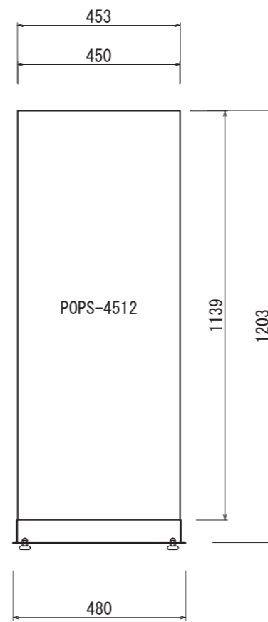
【正面図 S=1:15】
