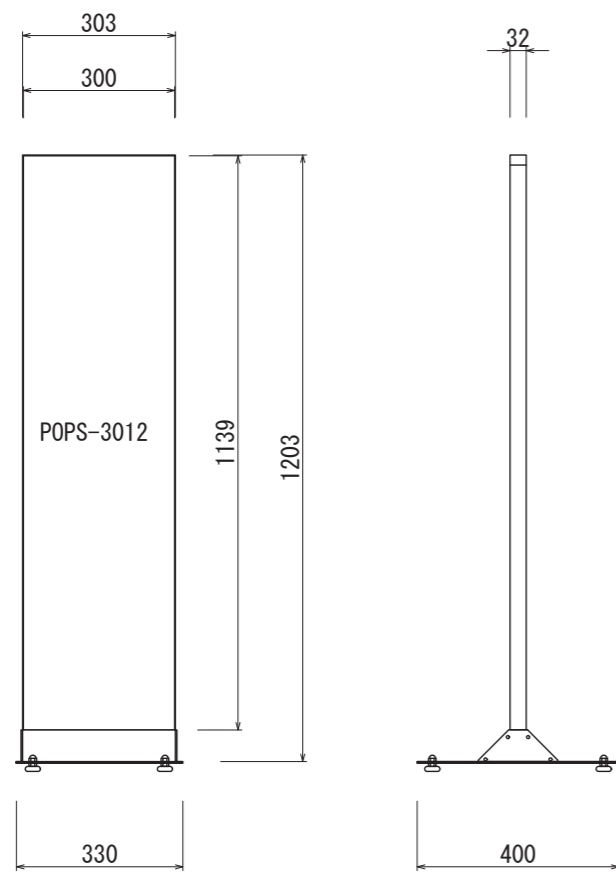
【正面図 S=1:15】
