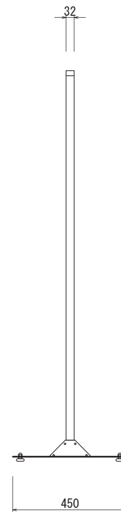
【側面図 S=1:15】
