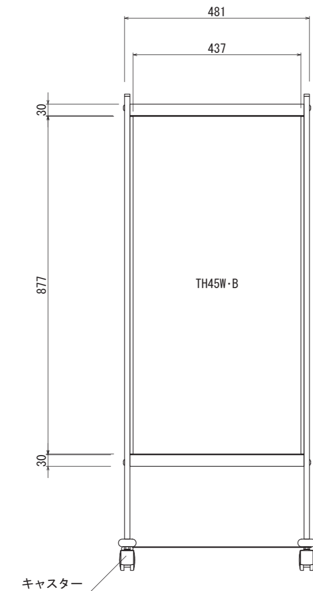
【正面図 S=1:10】
