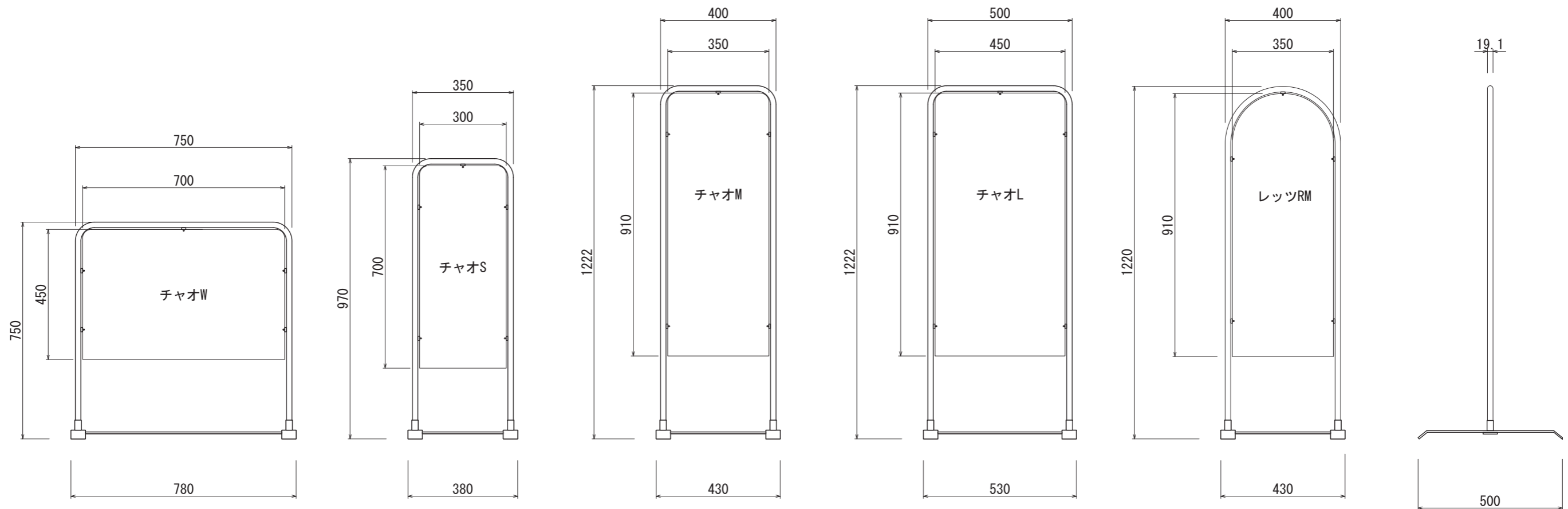
【正面図 S=1:15】
