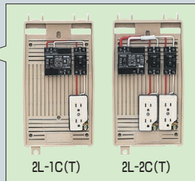
本体(WB-2LJ)
