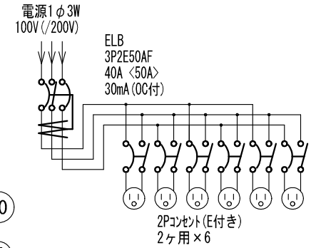
結線図
