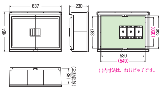
■WB-17AY□ ●木板ベース付
