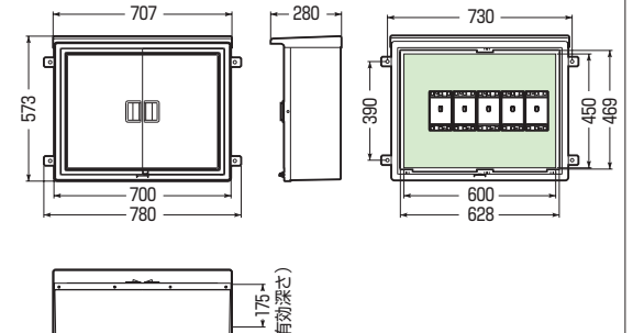
■WB-18A□ ●木板ベース付
