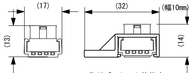
取付ブラケット装着時 側面拡大図
