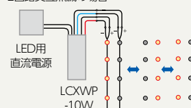
2回路交互点滅の場合
