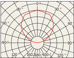
トキラックス 配光
